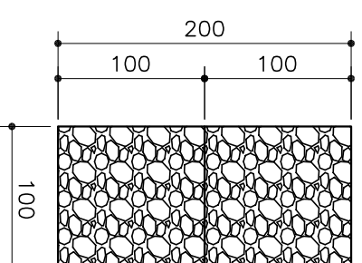
Detalhe Construtivo Gabião Ponte do Beco Extensão 12,00m
